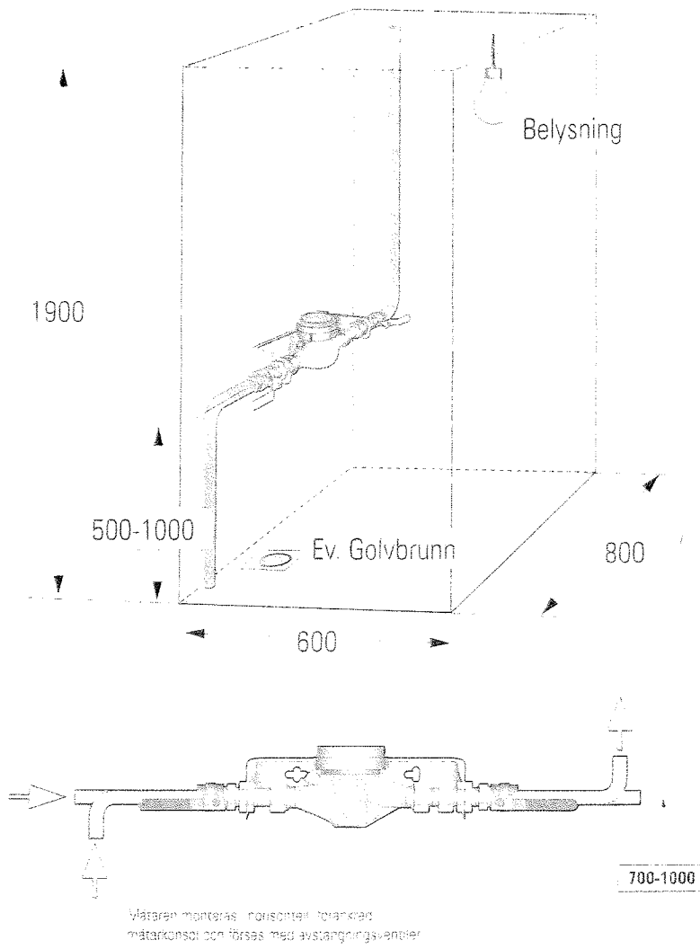
Figur 9.1 Vattenmätarplats.
